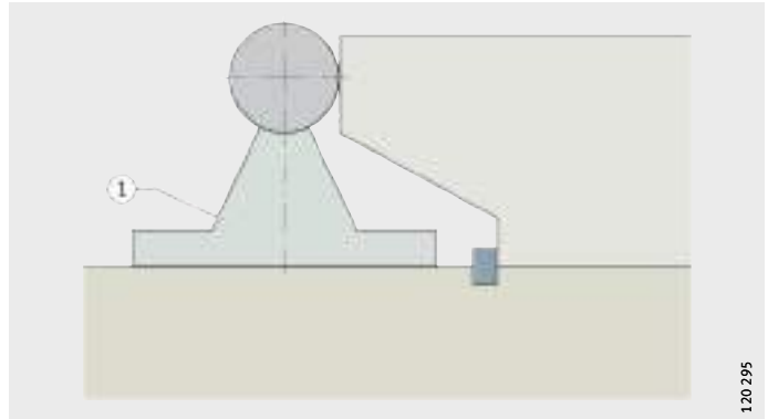
Figura 5 Alineación de un carril-soporte con el eje
